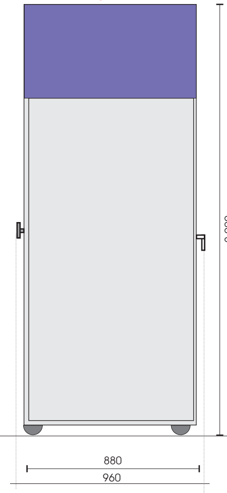
VISTA LATERALIZQUIERDA LEFT SIDE VIEW
