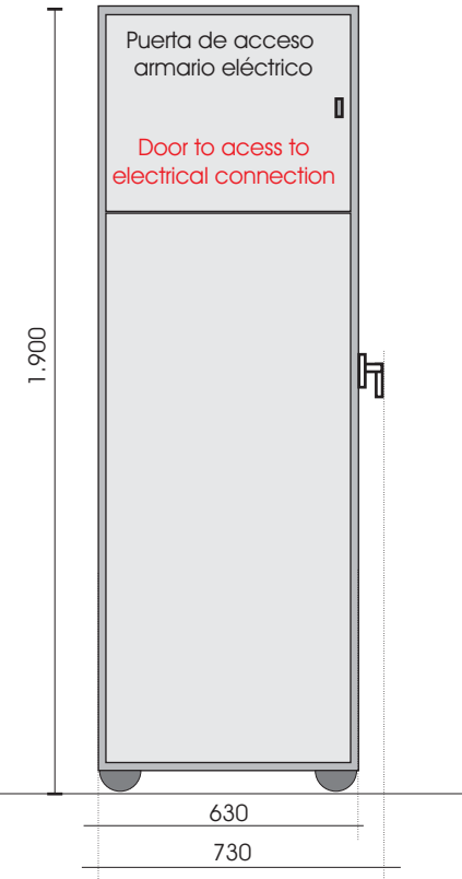
VISTA LATERALIZQUIERDA LEFT SIDE VIEW
